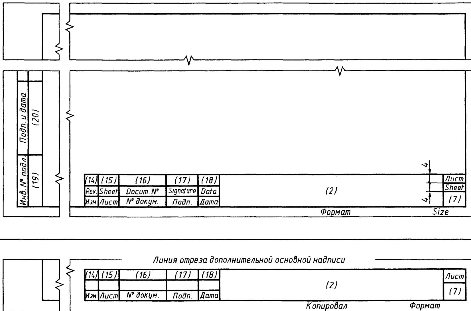
Форма 3 — Основная надпись для текстовых конструкторских документов (последующие листы)
