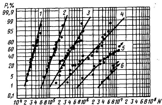
Кривые распределения долговечности образцов из сплава марки В95
