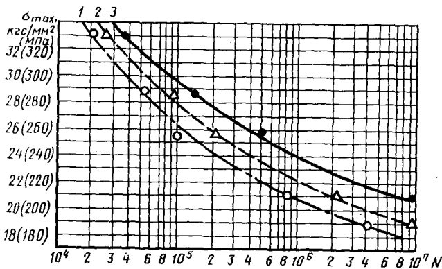
Кривые усталости образцов из сплава марки В95
