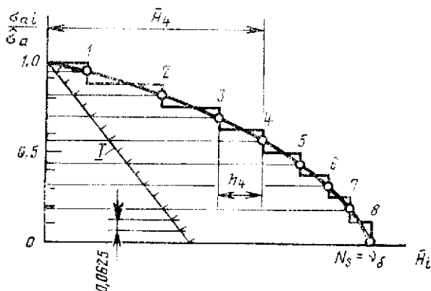
1—отрезок вспомогательной прямой, разделенный на 16 равных частей; 1—8—ступени блока.
